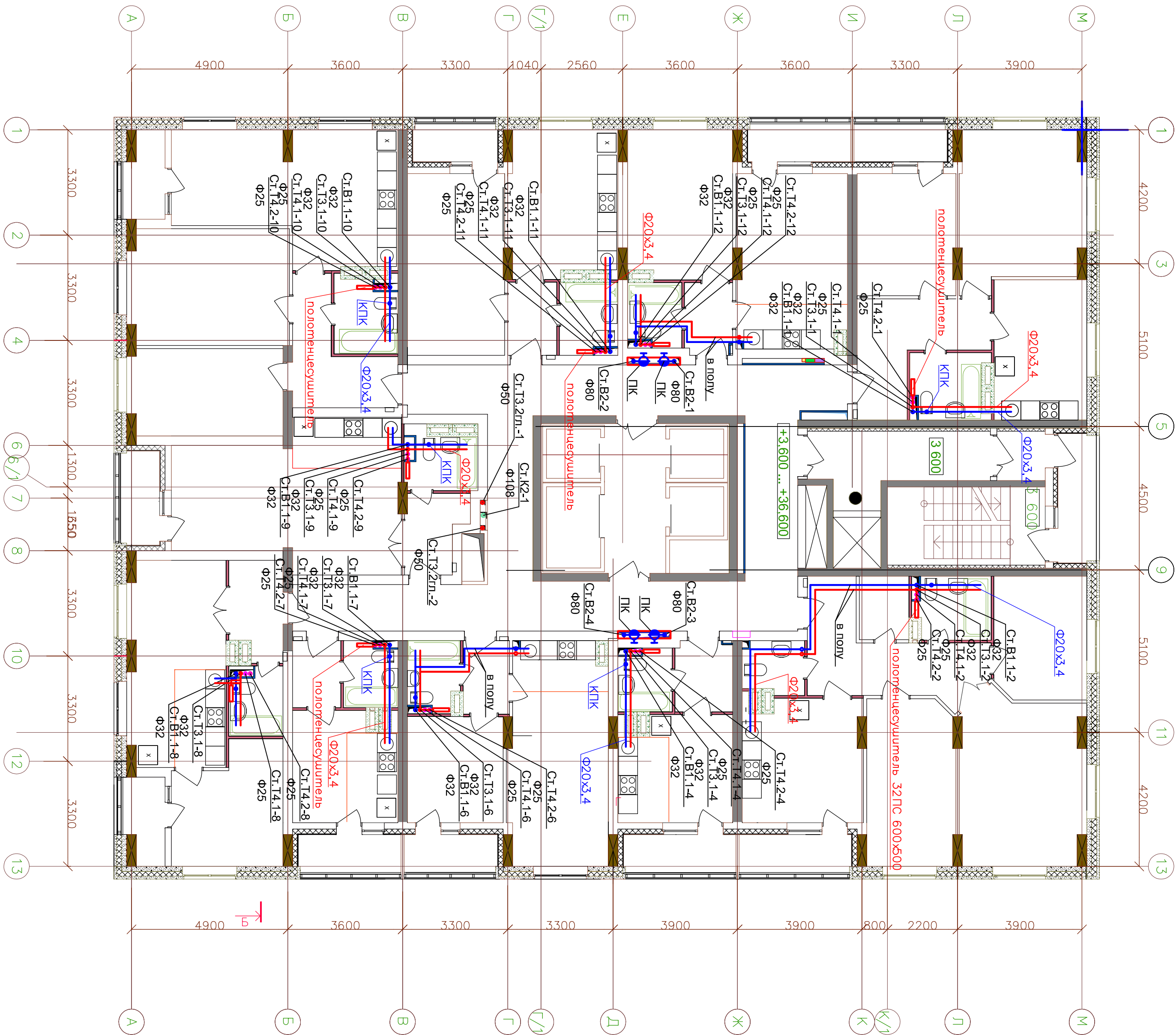
План 2-13 этажей с сетями В1.1, В2, Т3.1, Т3.2, Т4.1, Т4.2
